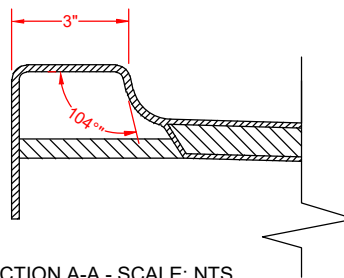
SECTION A-A - SCALE: NTS
