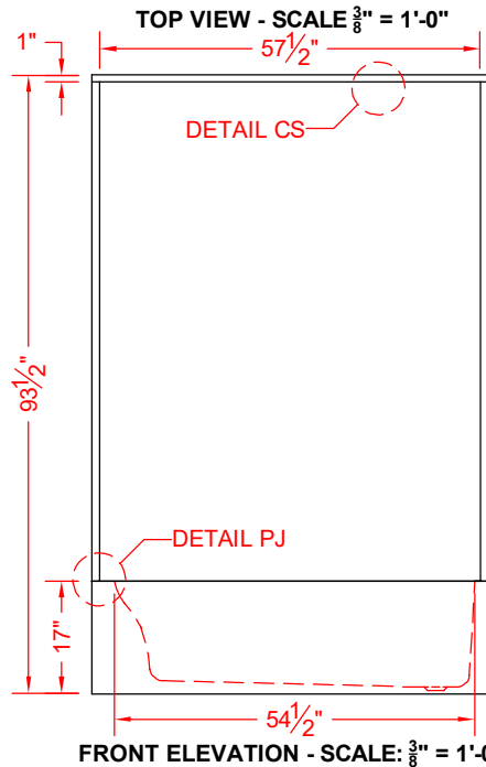
FRONT ELEVATION - SCALE: \frac{3}{8}'' = 1'-0''
